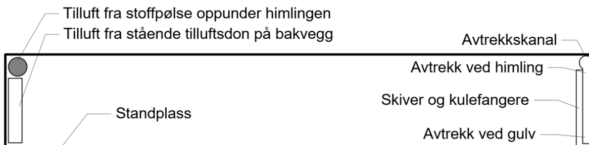
Figur 2 Prinsippkisse ventilasjon, vertikalsnitt i lengderetningen gjennom baneløpet
