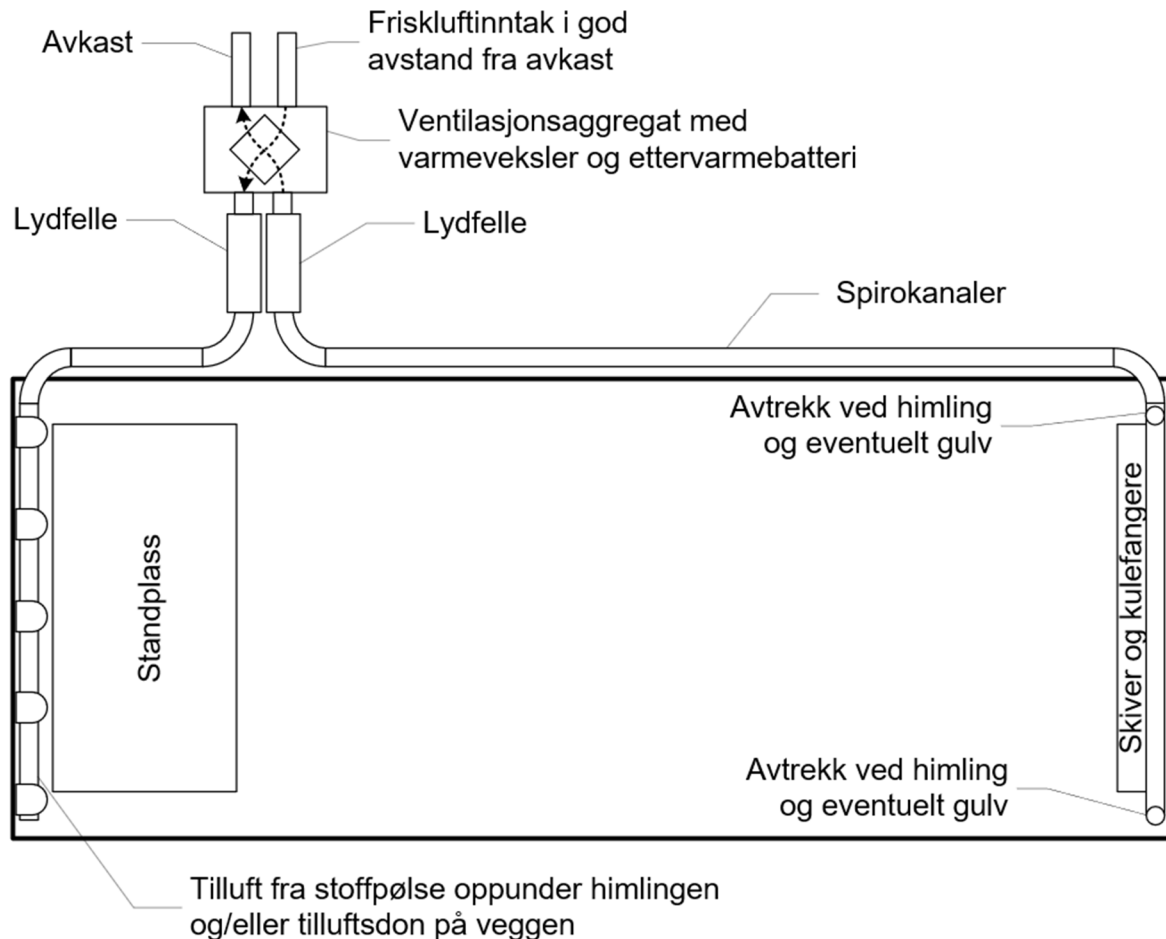
Figur 1 Prinsippkisse ventilasjon på plantegning
